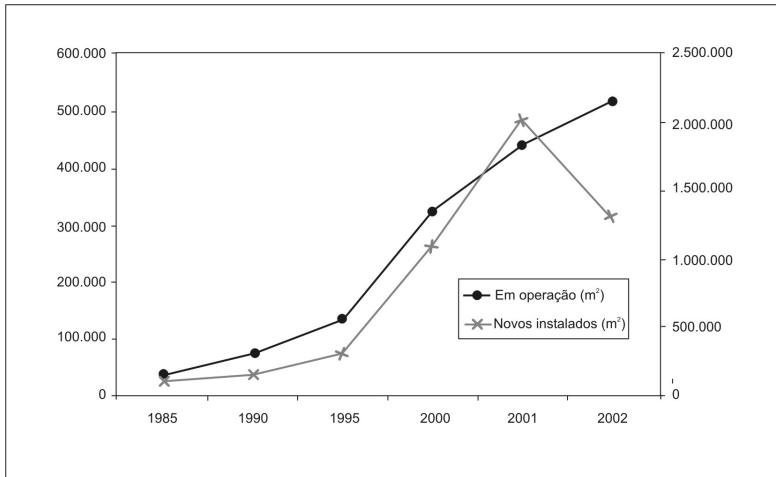
Figura 3. Produção anual e instalação acumulada de coletores solares – Brasil 15
