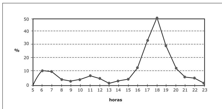
Figura 1. Uso do chuveiro elétrico ao longo do dia nas residências - região Sudeste, 1988
