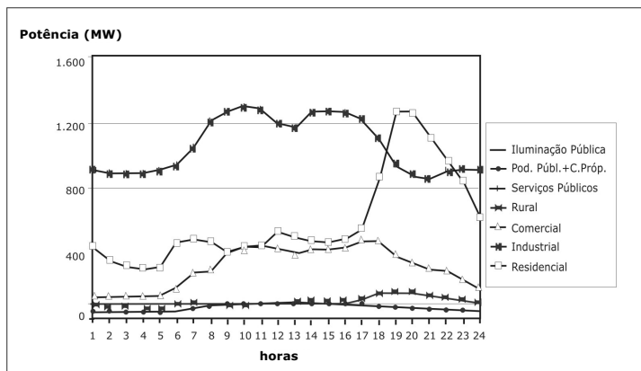
Figura 5. Desagregação da curva de carga do sistema CPFL – 2004
